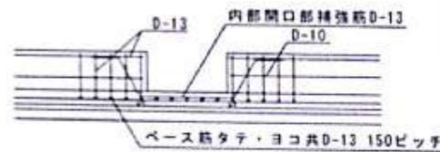
内部開口部補強筋詳細図
