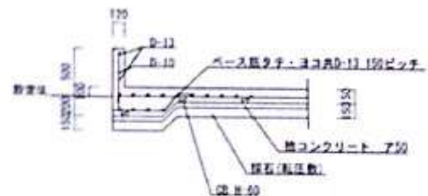
基礎断面詳細図
